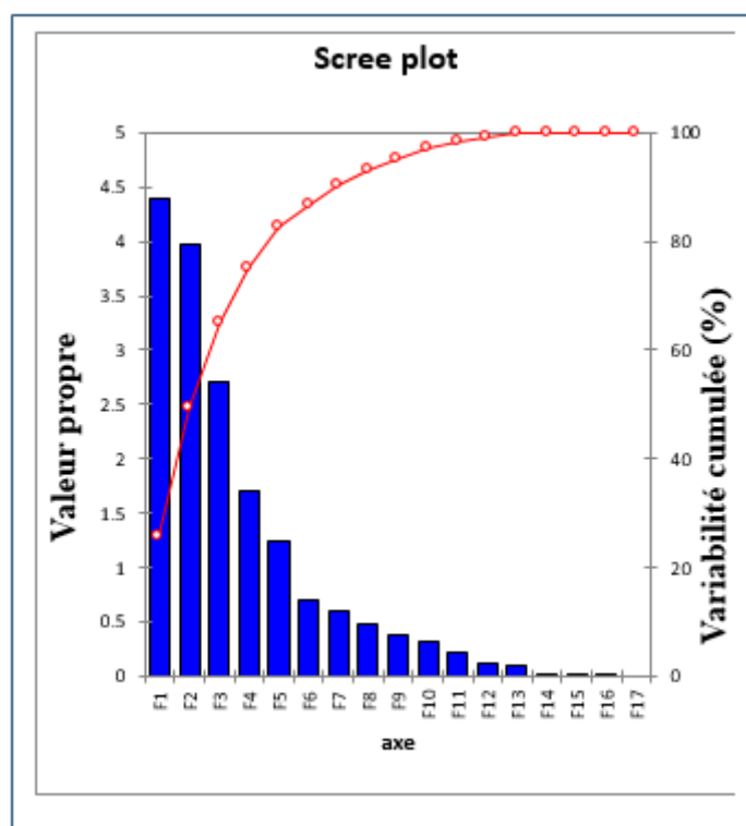
Figure 2 : graphe des valeurs propres
